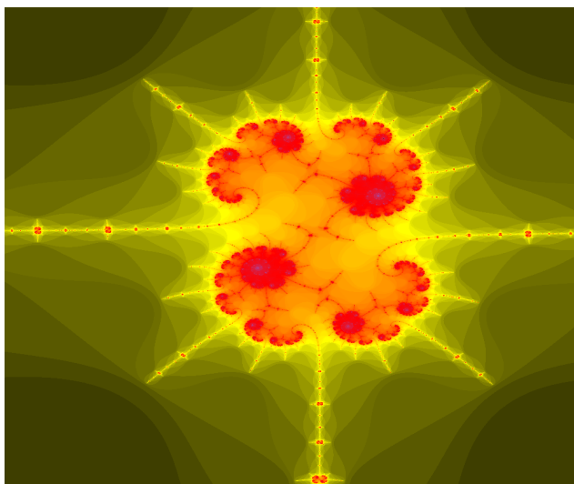
Juliova množina c = -1,74774 + 0,0009819i
