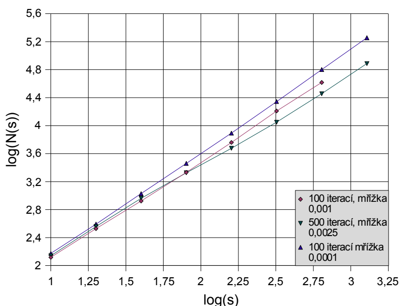
Obrázek 35 Log-log graf pro měření dimenze Mandelbroty množiny pro data z tabulek 8, 9 a 10.
