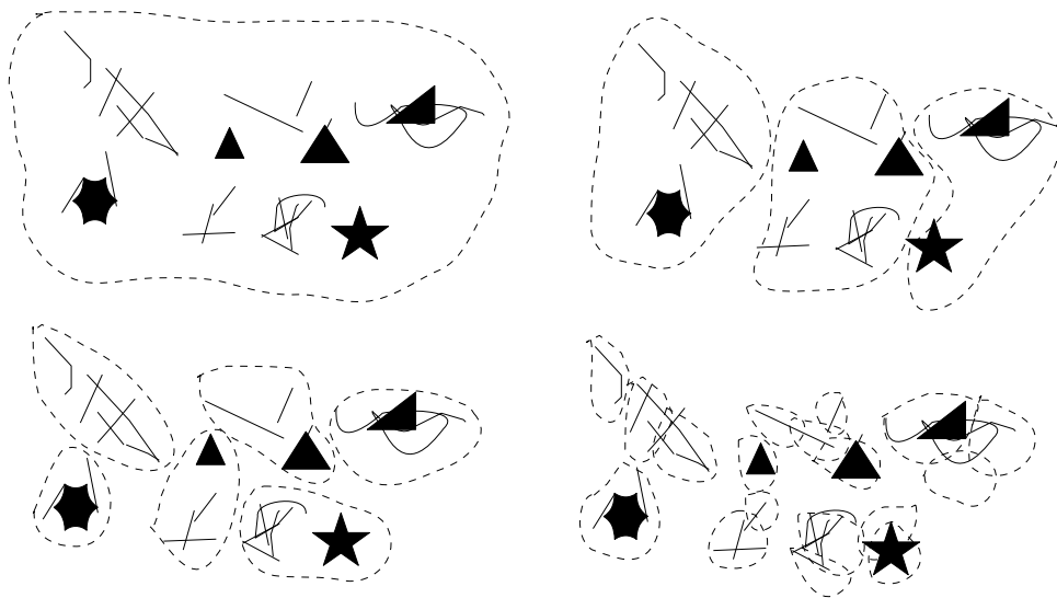
Obrázek 10 Různá pokrytí množiny pro zmenšující se \varepsilon .
