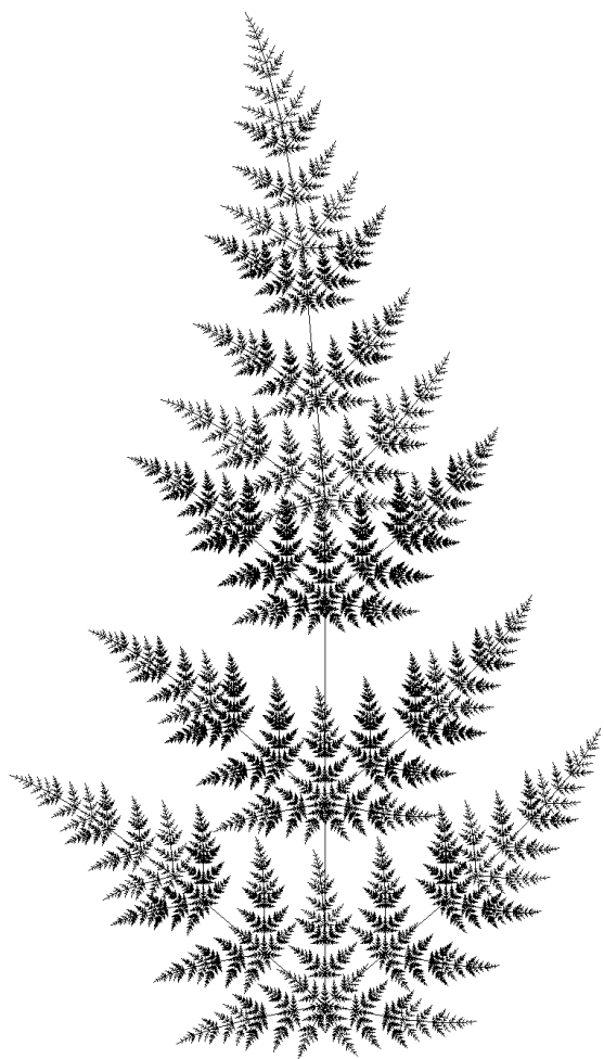
IFS kapradí
