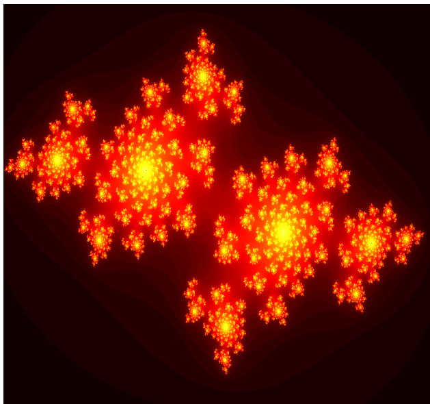
Obrázek 20 Juliova množina -0.7091 + 0.3160i
