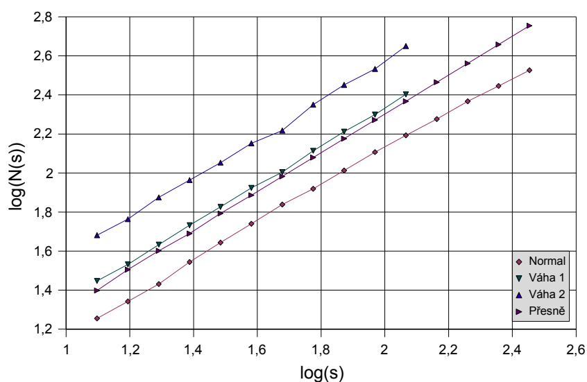
Obrázek 28 Mřížková dimenze úsečky
