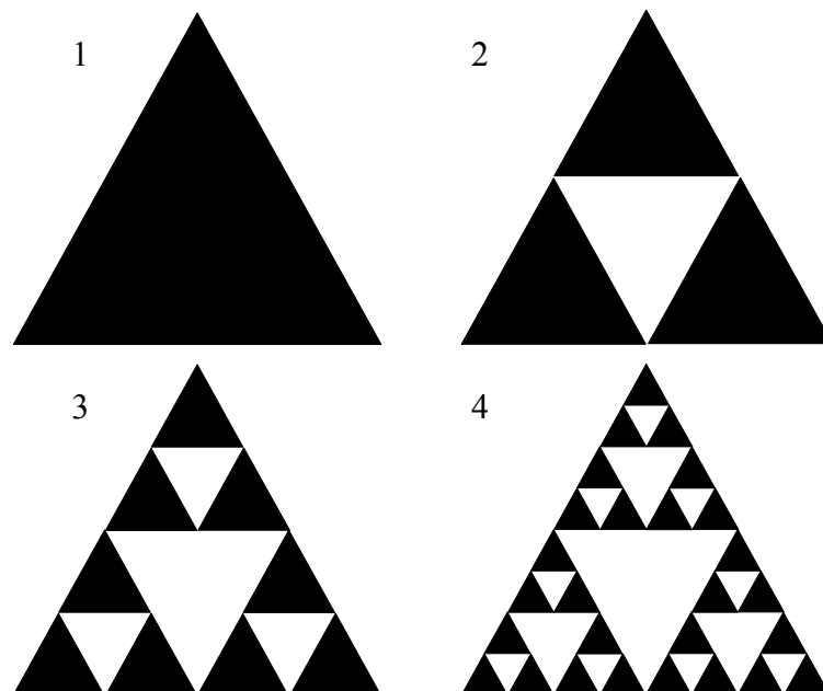
Obrázek 4 Konstrukce Sierpińského trojúhelníku
