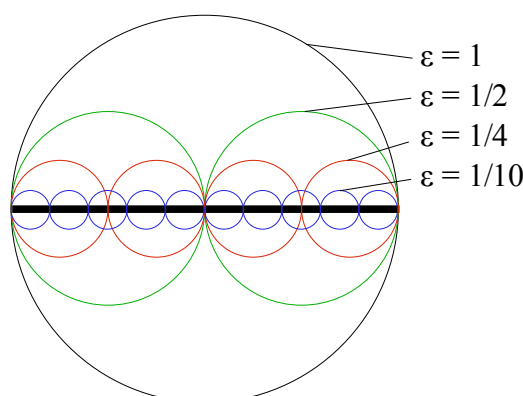
Obrázek 12 Pokrytí intervalu \langle 0, 1 \rangle
