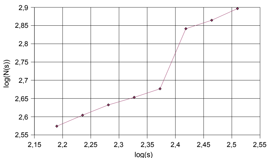
Obrázek 27 Chyba při nedostatečně jemnosti mřížky při použití vah buněk
