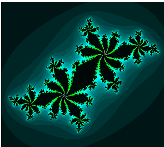
Obrázek 22 Juliova množina -0.3555 - 0.62007i
