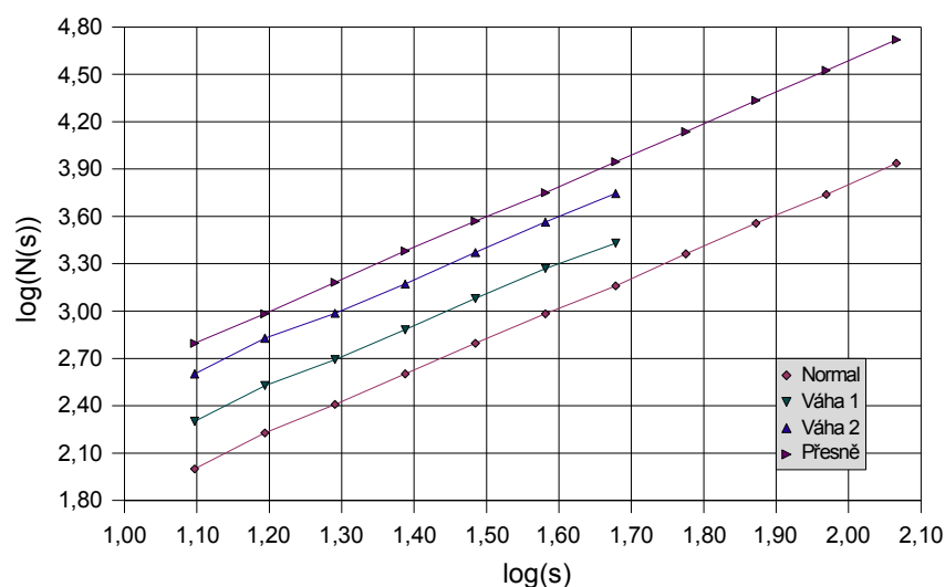
Obrázek 29 Mřížková dimenze čtverce
