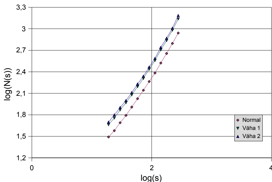
Obrázek 30 Mřížková dimenze úsečky tloušťky 5px
