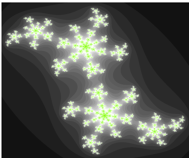
Juliova množina c = 0,156 - 0,672i
