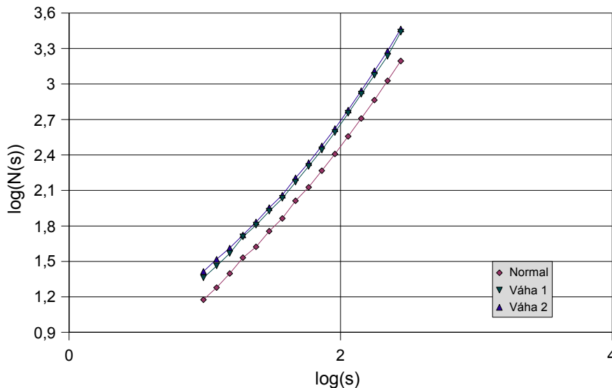
Obrázek 31 Mřížková dimenze úsečky tloušťky 10px
