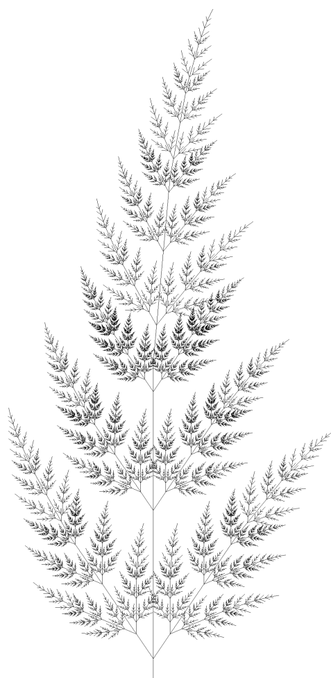
IFS kapradí
