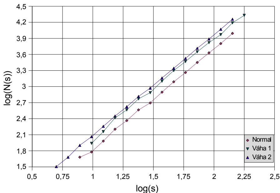
Obrázek 34 Mřížková dimenze Sierpiňského koberce
