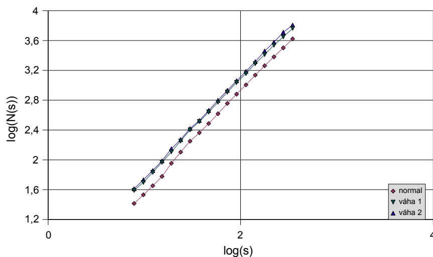
Obrázek 37 Log-log graf měření dimenze Mandelbrotovy množiny z rastrového obrázku.
