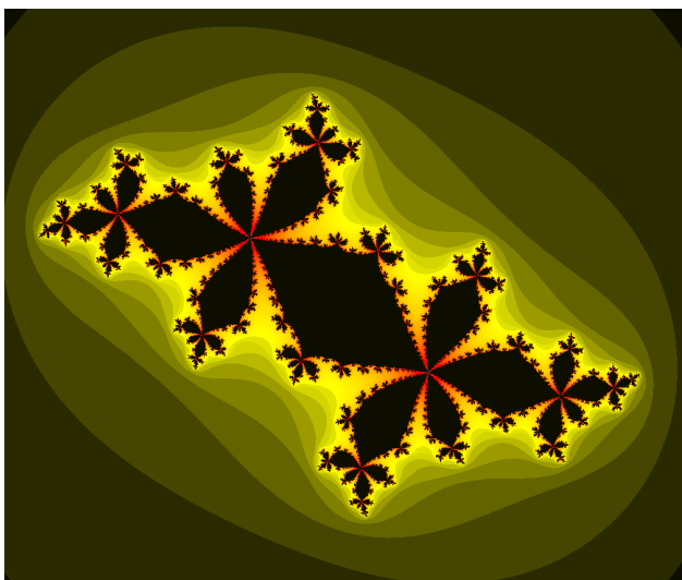
Juliova množina c = -0,505 + 0,565i
