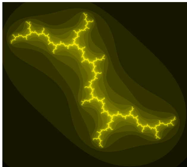
Obrázek 23 Juliova množina 0 + 1i
