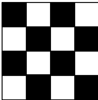
Obrázek 26 Započítání méně čtverců než je třeba
