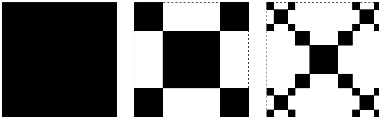
Obrázek 16 Konstrukce množiny
