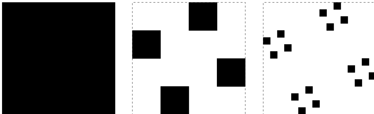
Obrázek 15 Konstrukce Cantorova diskontinua, \dim_H F = 1
