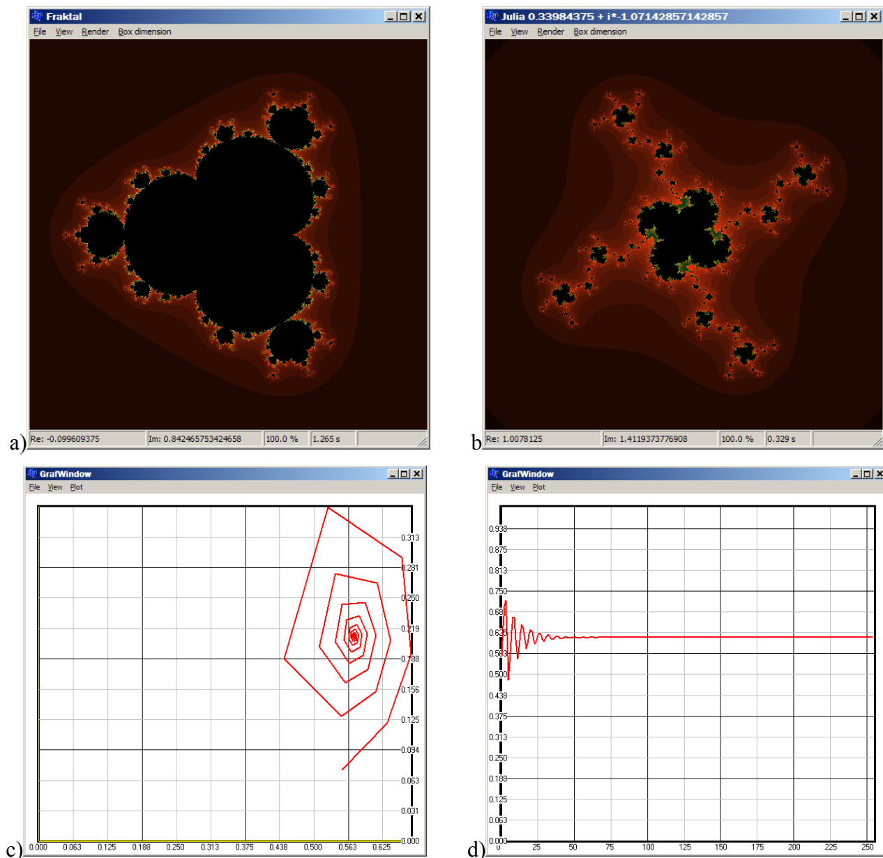
Obrázek 38 Program pro zobrazení a průzkum Mandelbrotovy množiny a Juliových množin.
