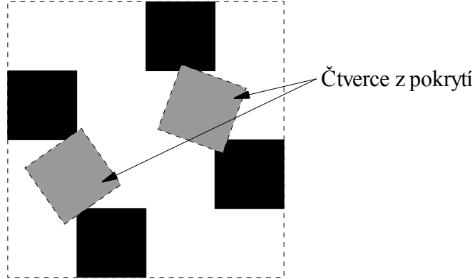
Obrázek 19 Dolní odhad mřížkové dimenze, čtverce z pokrytí protnou maximálně dva čtverce množiny F .
