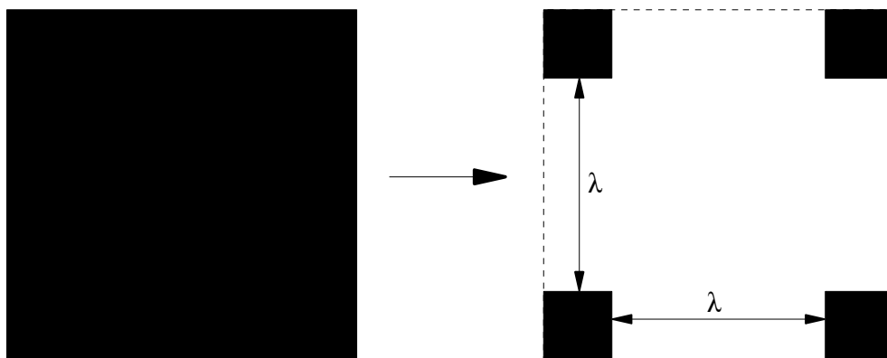
Obrázek 18 Postup pro vytvoření množiny F \times F , kde F je upravená Cantorova množina
