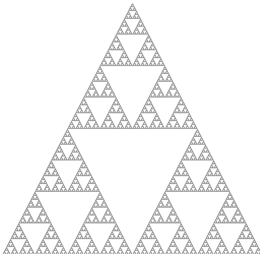
Sierpińského trojúhelník
