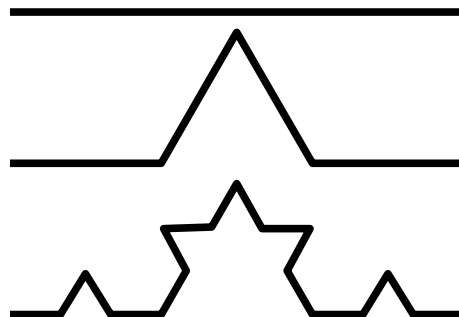
Obrázek 2 Konstrukce Kochovy křivky
