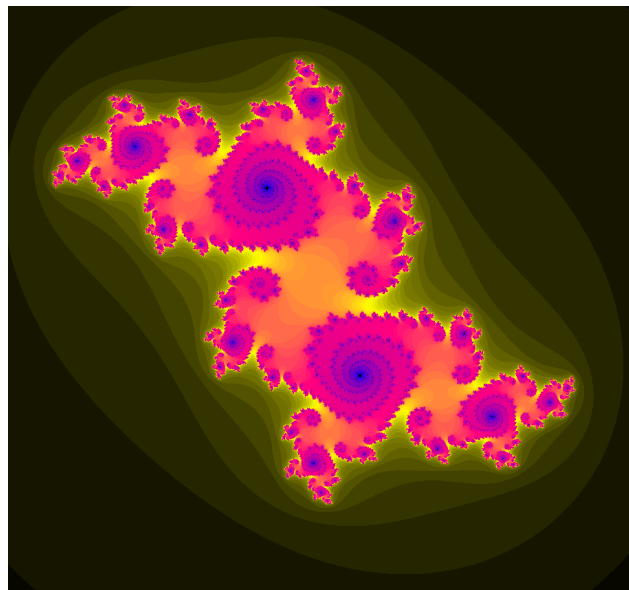
Obrázek 21 Juliova množina -0.0585 + 0.66i
