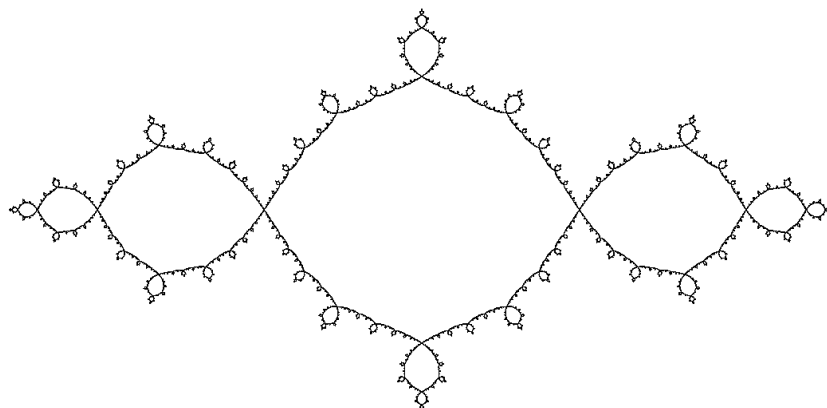
Obrázek 6 Hranice Juliovy množiny pro c = 1 + 0i
