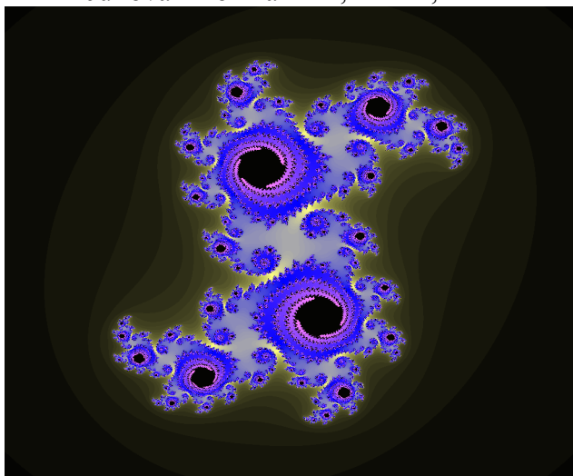
Juliova množina c = 0,363443 + 0,31565i
