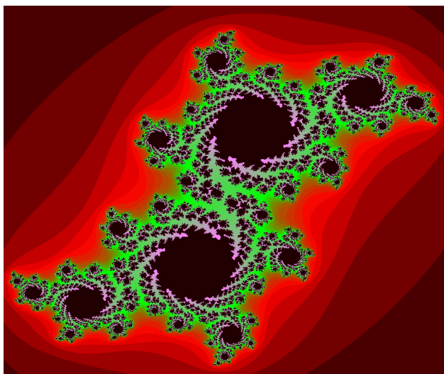
Juliova množina c = 0,060124 - 0,62422i
