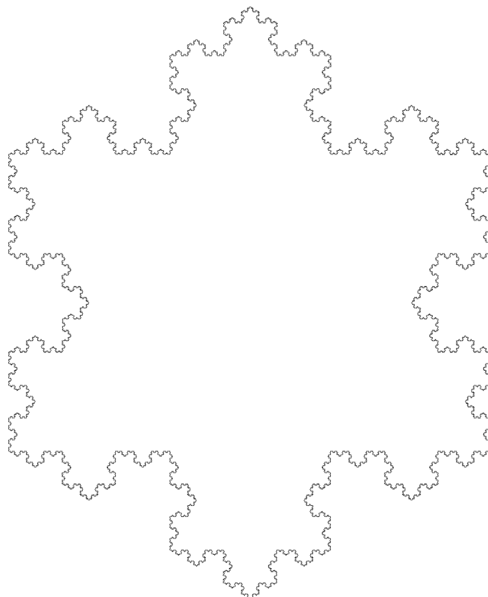
Kochova vločka
