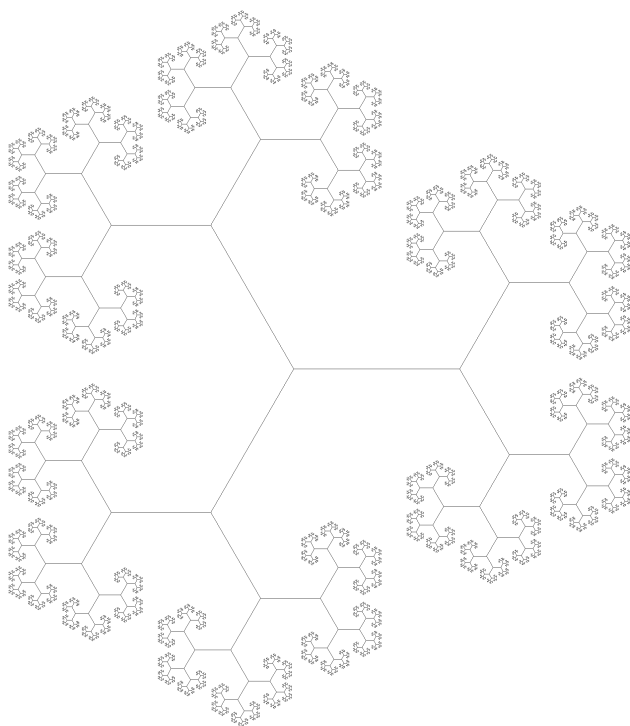
IFS květák
