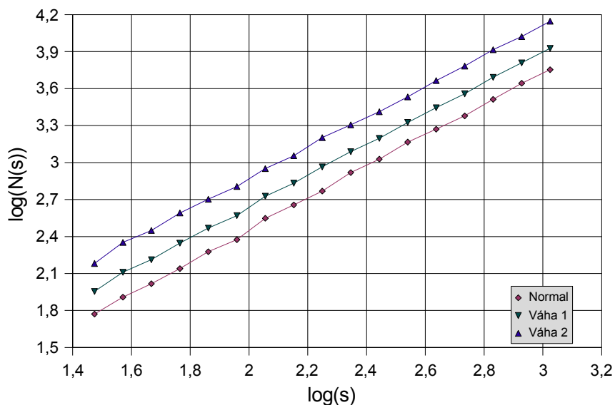
Obrázek 32 Mřížková dimenze Kochovy křivky
