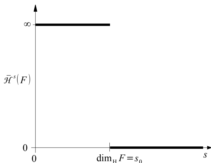
Obrázek 11 Hodnota Hausdorffovy míry v závislosti na s
