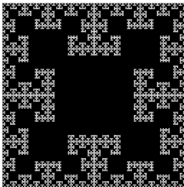
IFS koberec
