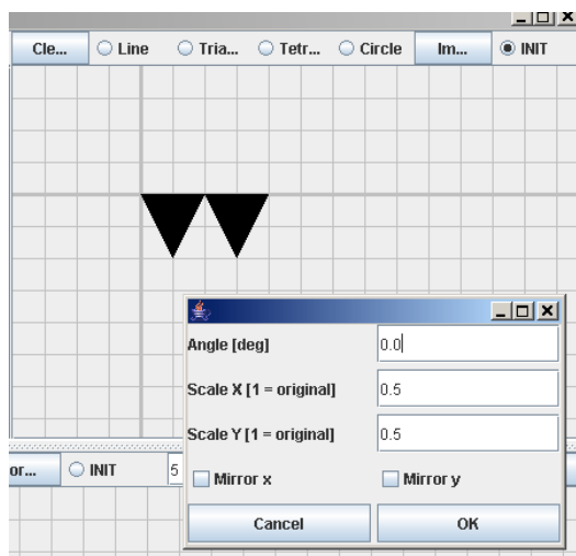
Obrázek 41 Kreslení generátoru
