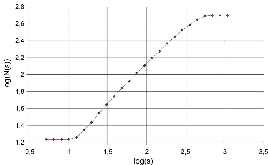
Obrázek 24 Log-log graf při měření mřížkové dimenze
