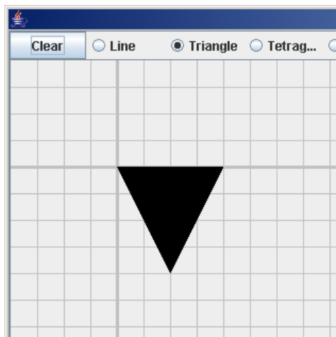
Obrázek 40 Kreslení iniciátoru
