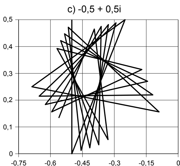
Obrázek 9 Iterační posloupnosti pro různé body Mandelbroty množiny.
