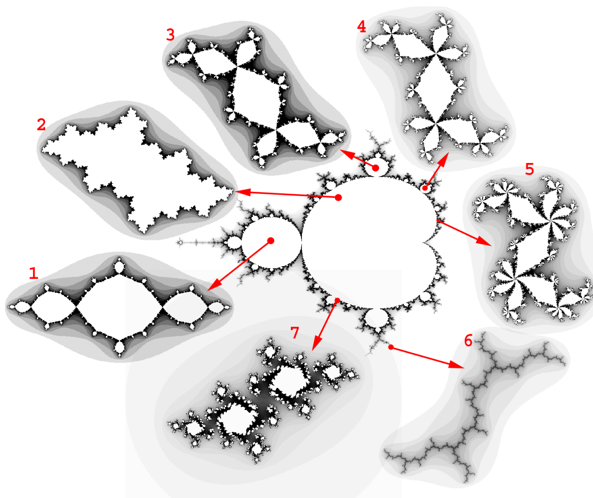
Obrázek 8 Ukázky Juliovy množiny v závislosti na pozici v Mandelbrotově množině.
