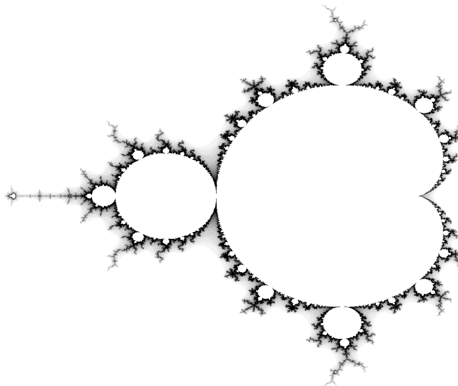
Obrázek 7 Mandelbrotova množina
