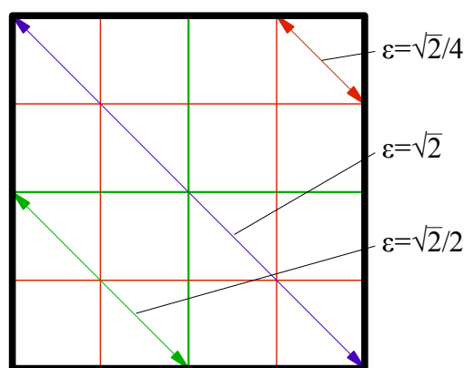
Obrázek 13 Pokrytí jednotkového čtverce
