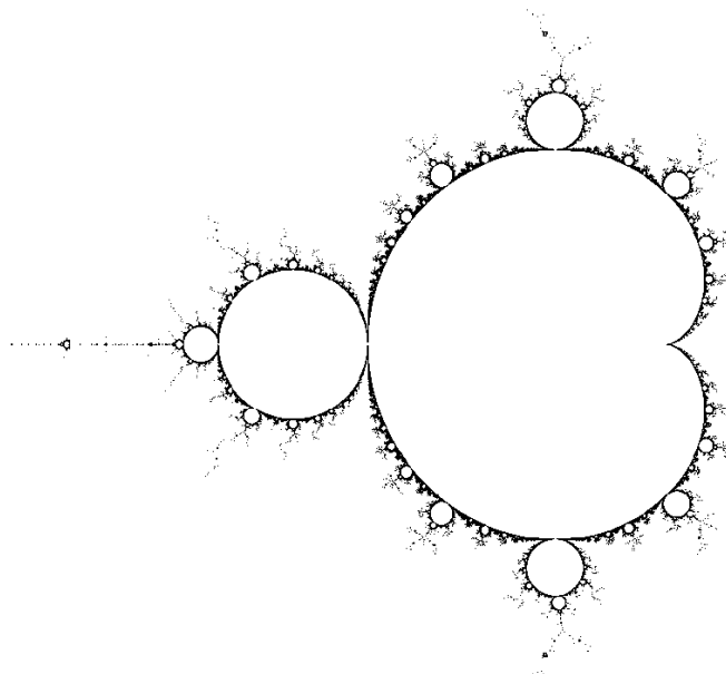
Obrázek 36 Rastrová verze Mandelbrotovy množiny použitá pro měření
