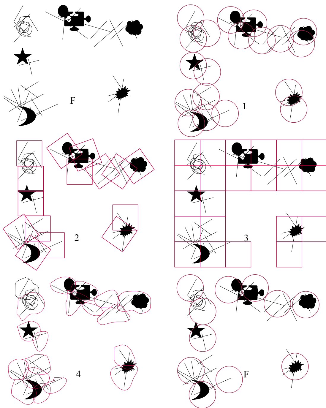
Obrázek 14 Pět způsobů, jak najít mřížkovou dimenzi množiny. Obrázky odpovídají bodům ve větě 17. Hodnota N_\delta(F) je tedy v prvním případě (1) nejmenší počet koulí s poloměrem \delta , v druhém případě (2) nejméně krychlí se stranou \delta , ve třetím (3) je to počet krychlí z mřížky o straně \delta , které protínají F , ve čtvrtém (4) nejméně množin s diametrem \delta a v pátém (5) je to největší počet disjunktních koulí s poloměrem \delta se středy v množině F .
