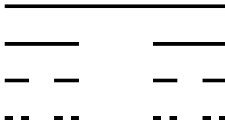
Obrázek 1 Konstrukce Cantorovy množiny
