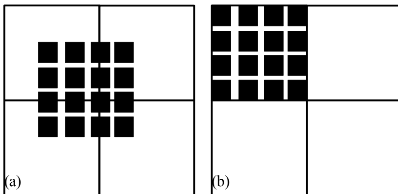
Obrázek 25 Příklad započítání více čtverců, než je třeba, (a) špatně, (b) správně
