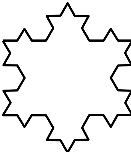
Obrázek 3 Kochova vložka nebo Kochův ostrov. Je získán tak, že místo úsečkou začneme rovnostranným trojúhelníkem
