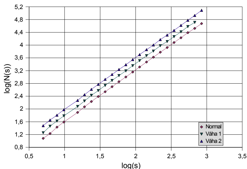
Obrázek 33 Mřížková dimenze Sierpiňského trojúhelníku
