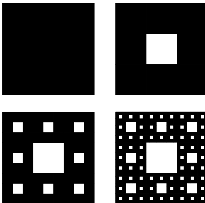
Obrázek 5 Konstrukce Sierpińského koberce
