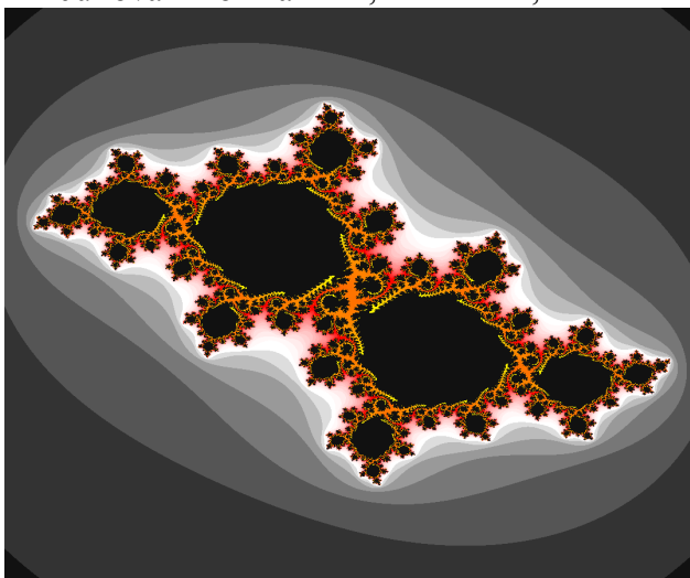
Juliova množina c = -0,401606 - 0,5819i
